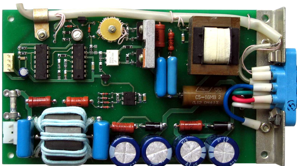
Рис. 2.7.1 Блок вращения анода RB07
