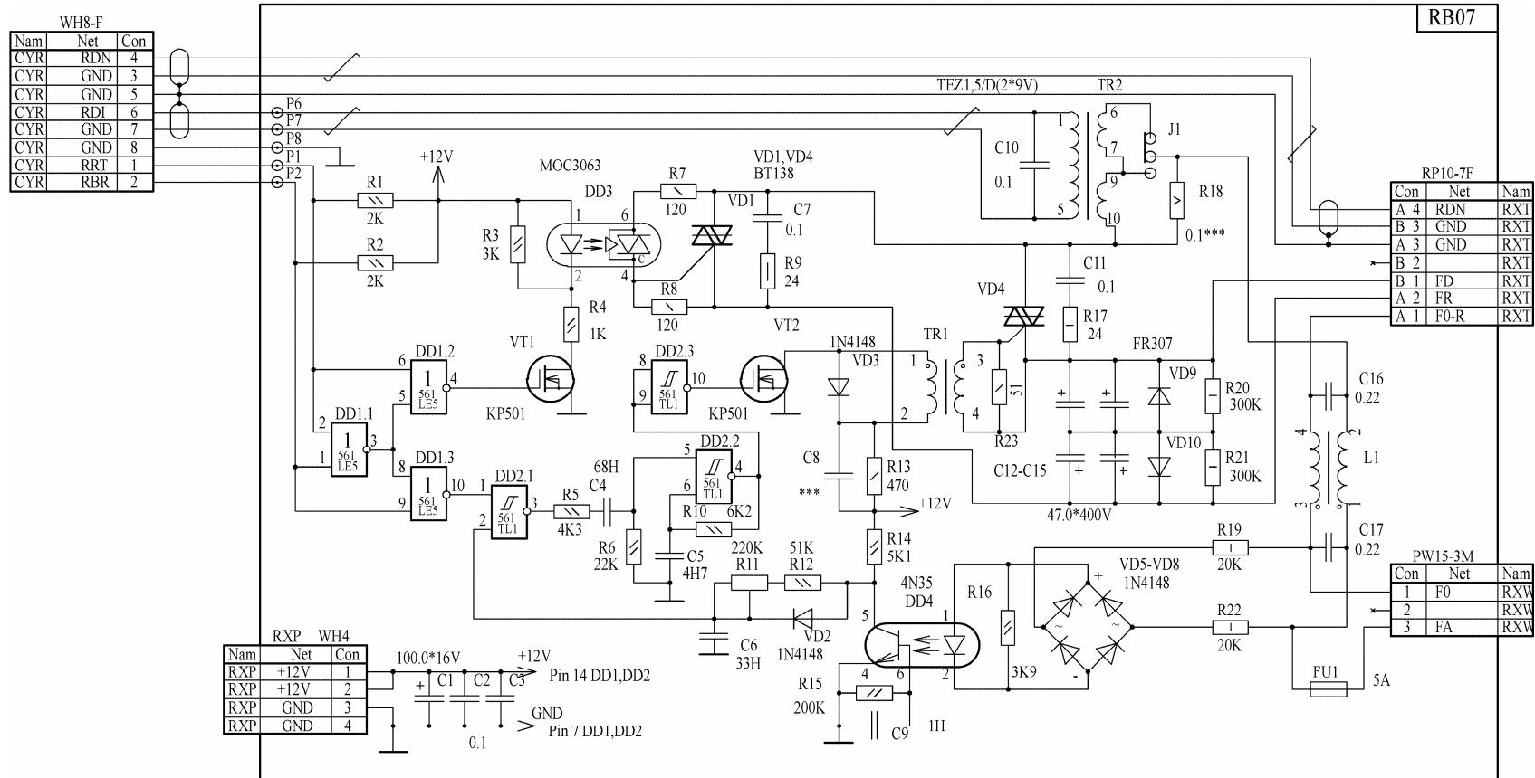
Рис. 2.7.2 Блок вращения анода RB07. Схема электрическая принципиальная
