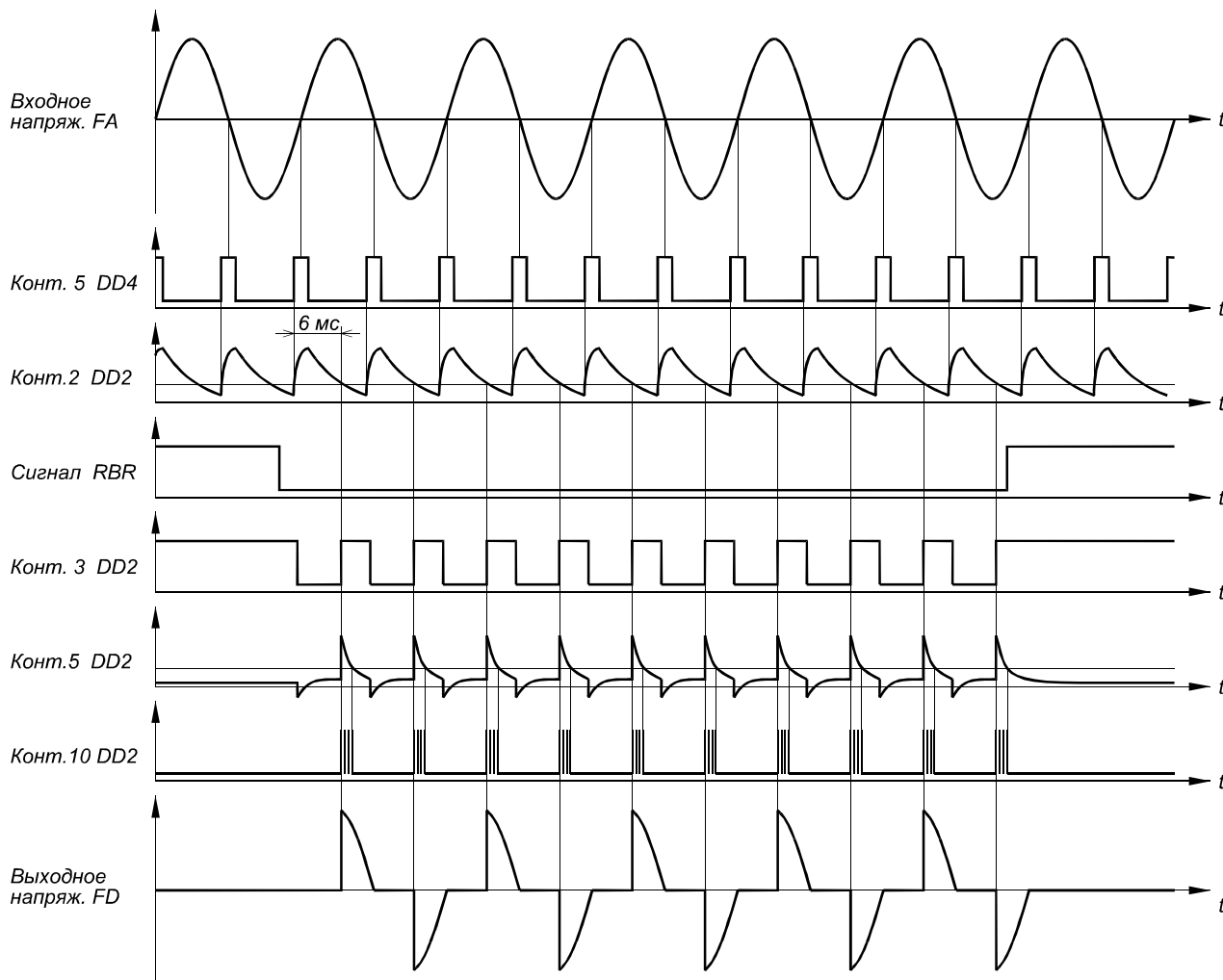
Рис. 2.7.4 Временные диаграммы сигналов в режиме торможения
