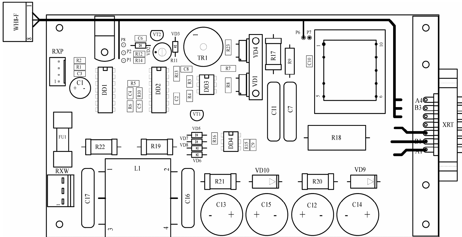
Рис. 2.7.3 Блок вращения анода RB07. Схема расположения элементов
