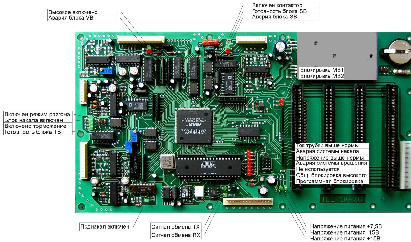
Рис 2.11.4. Органы световой индикации контроллера CR07.
