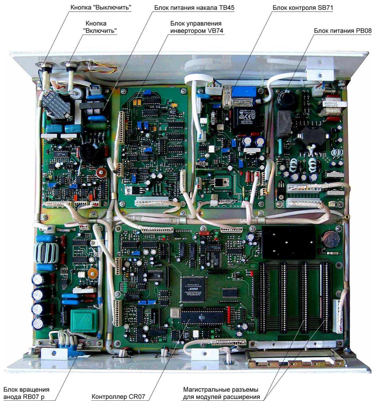
Рис. 2.1.2 Блок управления IEC-F7 со снятыми крышками кожуха. Вид сверху
