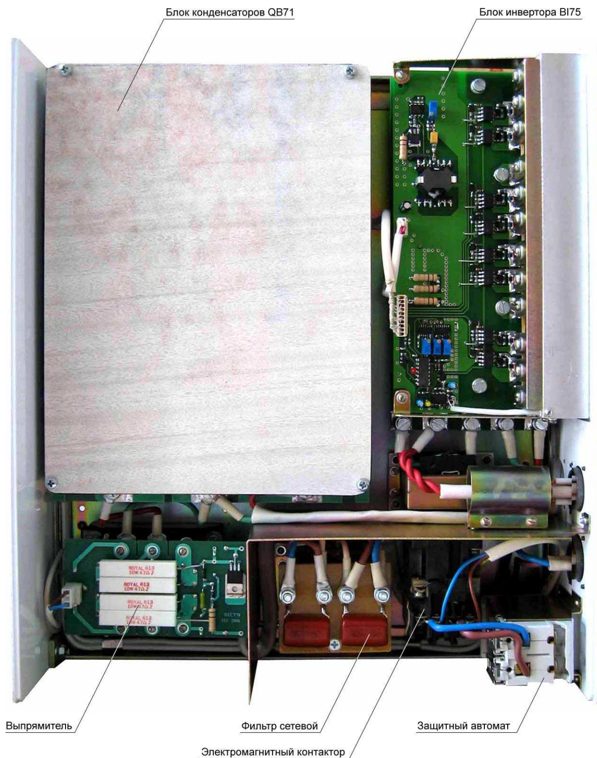
Рис. 2.1.3 Блок управления IEC-F7 со снятыми крышками кожуха. Вид снизу
