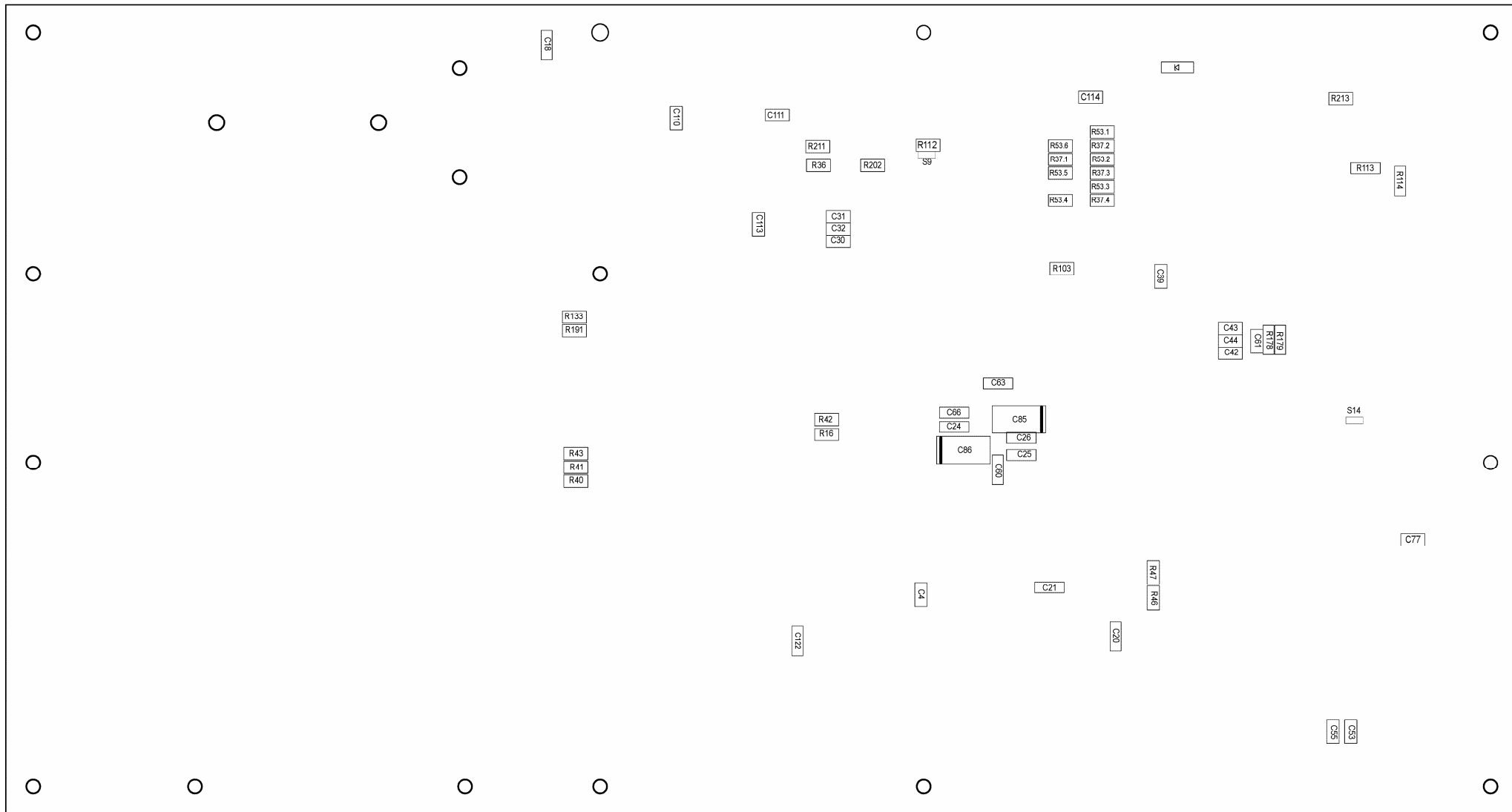
Рис. 2.11.7. Модуль CR-07. Схема расположения планарных элементов. Вид снизу
