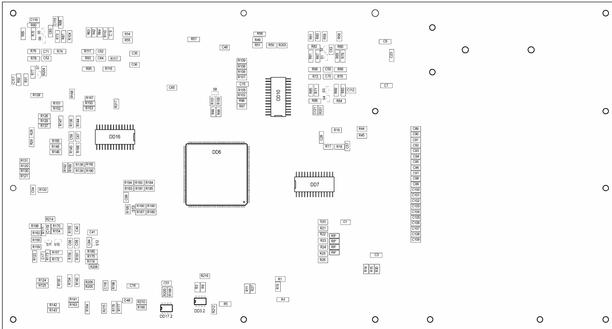
Рис. 2.11.7. Модуль CR-07. Схема расположения планарных элементов. Вид сверху
