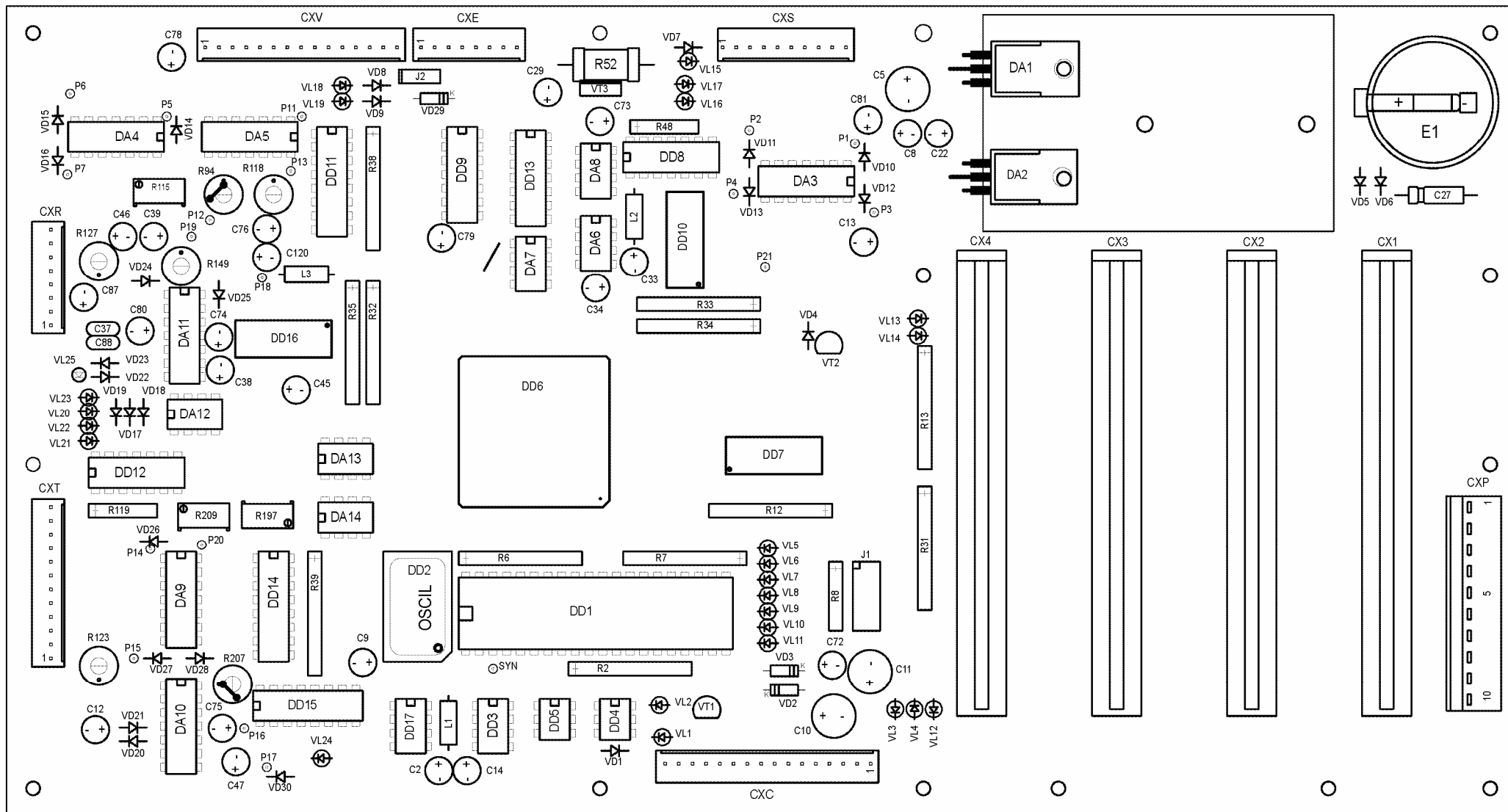
Рис. 2.11.6. Модуль CR-07. Схема расположения штыревых элементов
